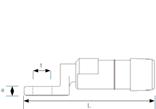
Изолированный наконечник с приваренным стержнем
