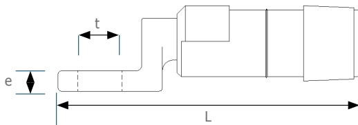
Изолированный наконечник с приваренным стержнем
