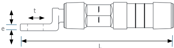
Изолированный опрессованный наконечник
