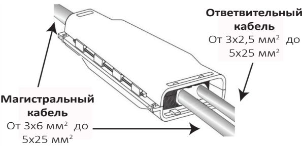
Разветвительная муфта
