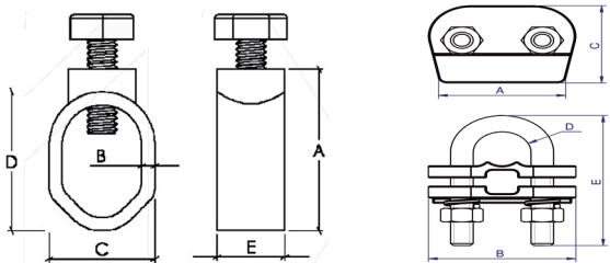
U-образный соединительный зажим F224
